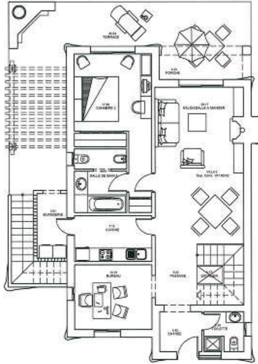
PLANTA BAJA ESC. 1/100
