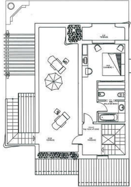
PLANTA ALTA ESC. 1/100
